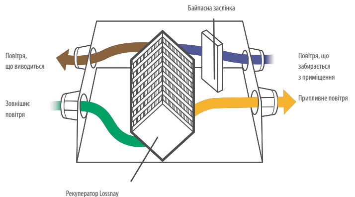
Байпасний режим
