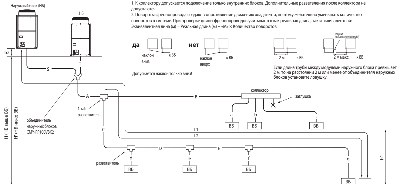
Рис. 6-1Б. Схема фреоновых проводов
