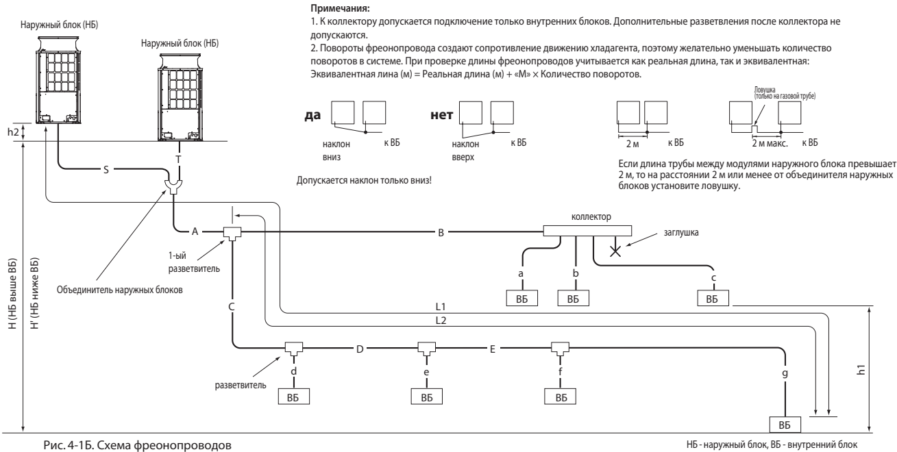
Рис. 4-1Б. Схема фреопроводов
