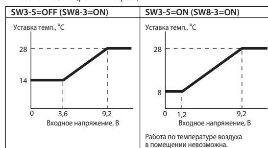
Рис. 4. Зависимость уставки температуры от управляющего сигнала
