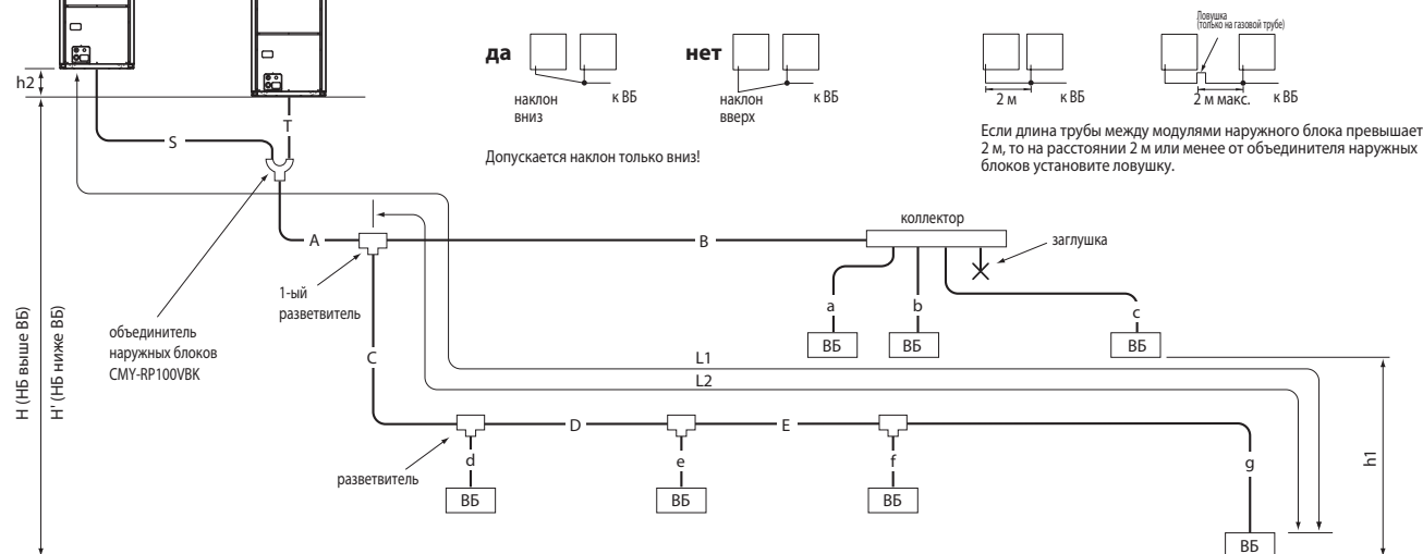
Рис. 6-1В. Схема фреоноводов
