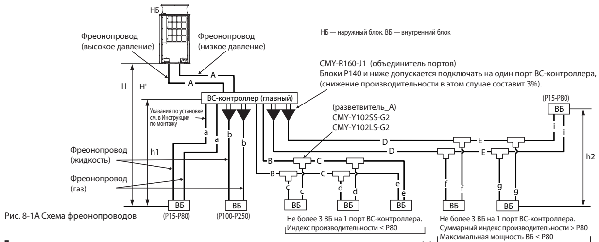
Рис. 8-1А Схема фреонопроводов
