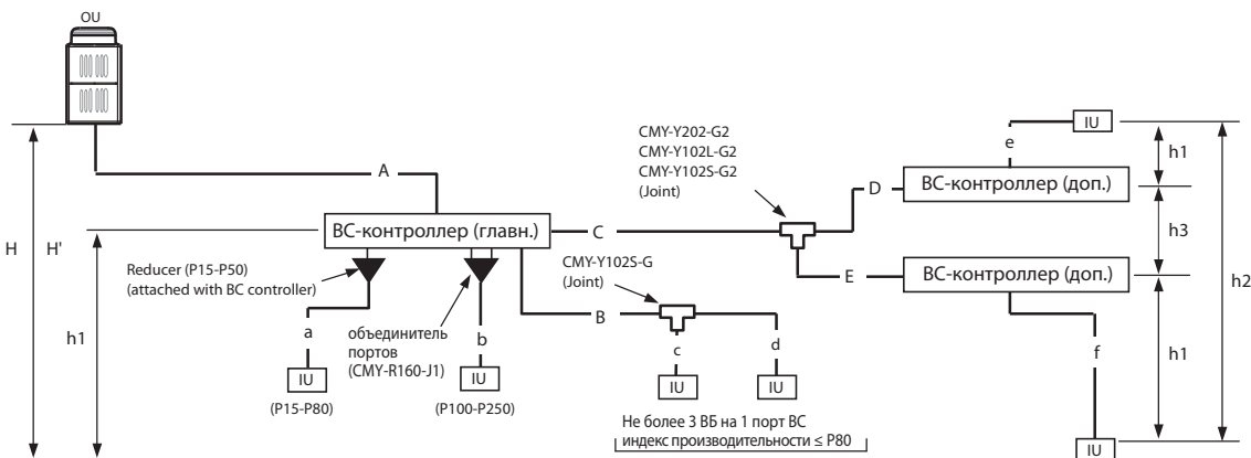
Рис. 10-2-2. Схема фреопроводов
