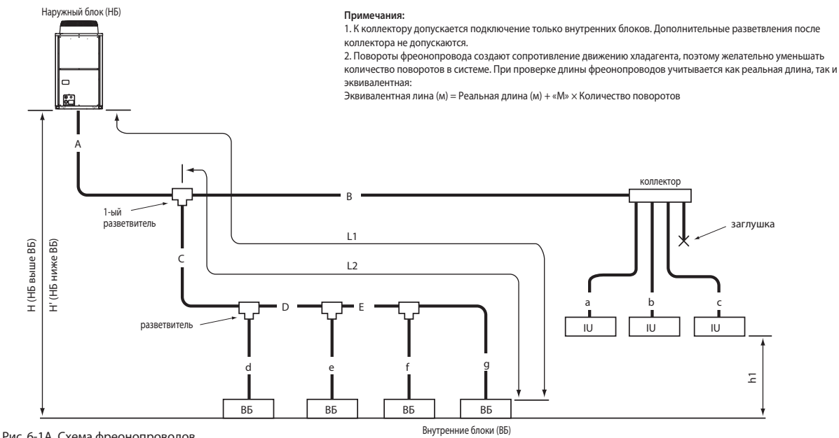
Рис. 6-1А. Схема фреопроводов
