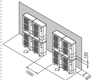
Рис. 4-10 Параллельное одиночное расположение
