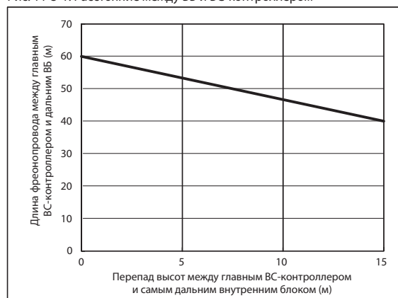
Рис. 11-3-1. Расстояние между ББ и ВС-контроллером
