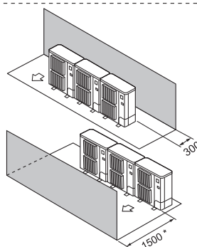
Рис. 4-7 Препятствие только сзади или спереди
