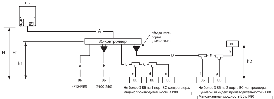
Рис. 11-2-1А. Схема фреонопроводов
