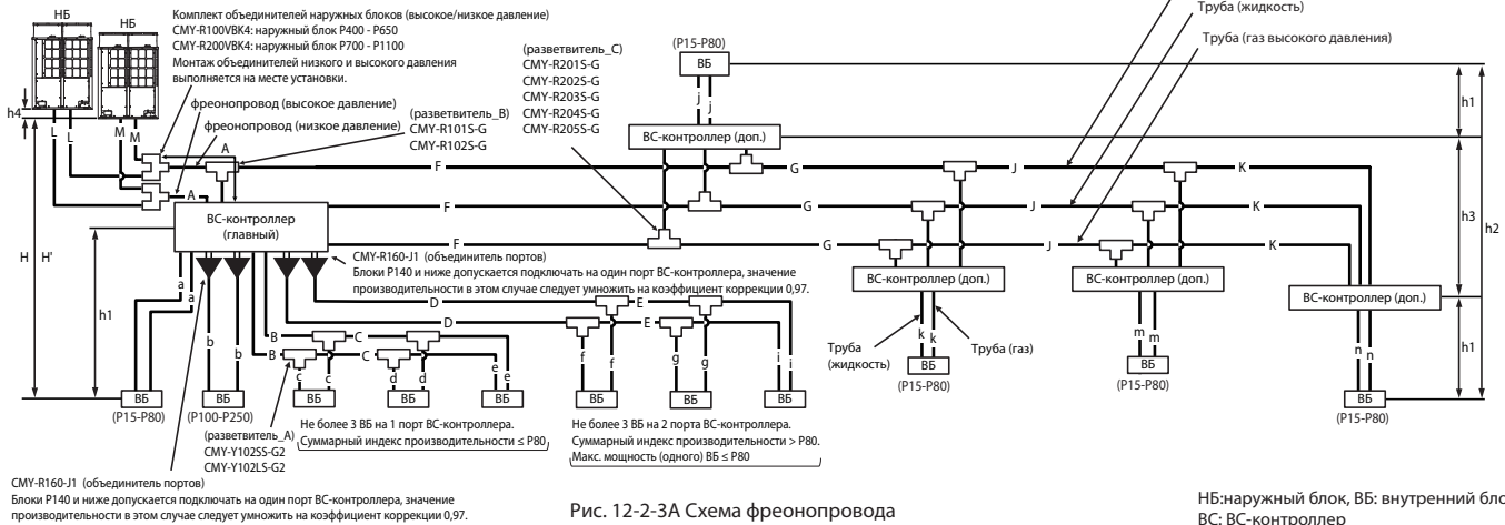
Рис. 12-2-3А Схема фреоновода
