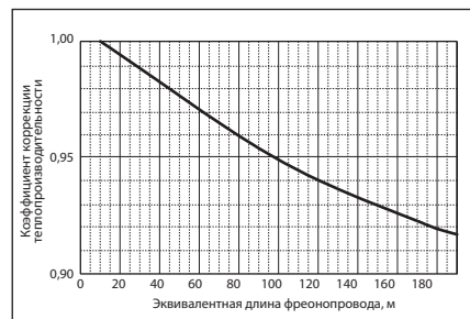
Рис. 6. Коррекция по длине фреонпровода
