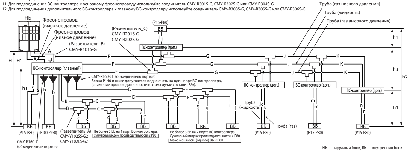
Рис. 8-1Б. Схема фреоноводов
