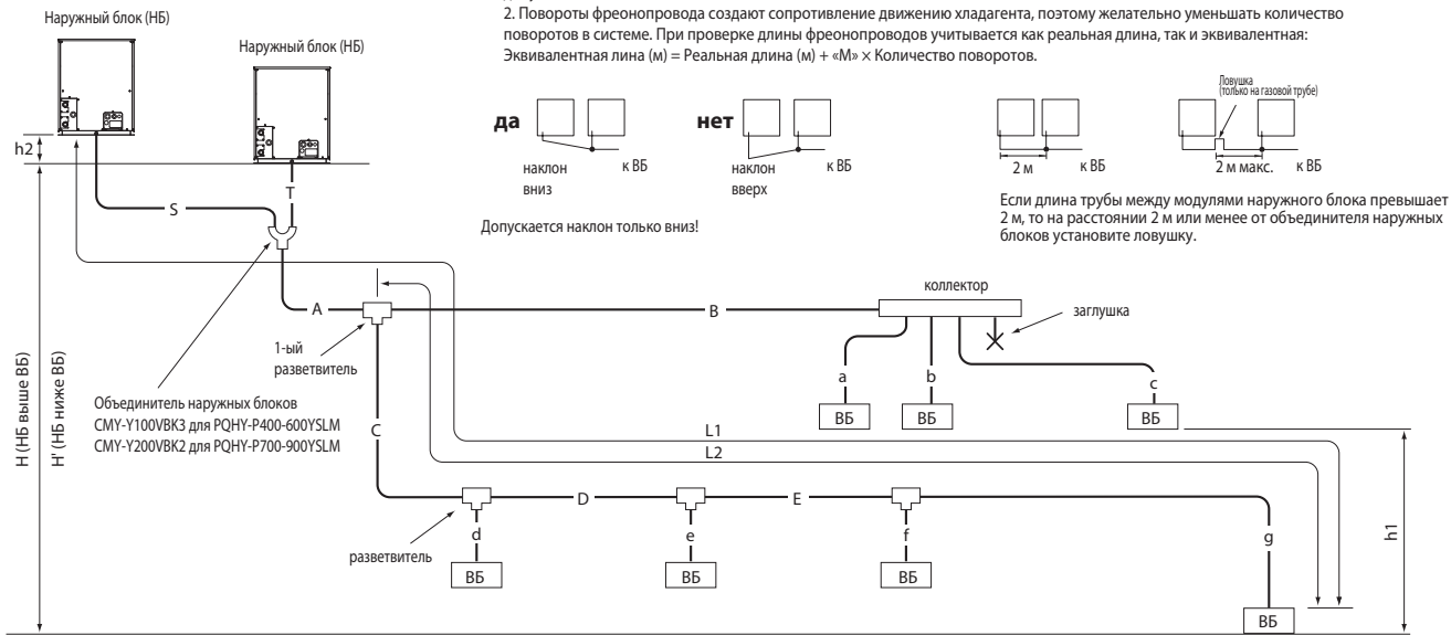
Рис. 7-1Б. Схема фреоноводов
