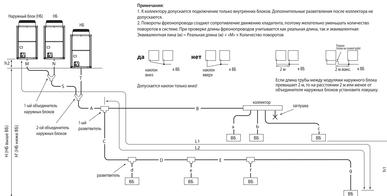
Рис. 6-1Г. Схема фреоноводов
